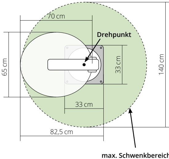
max. Schwenkbereich
